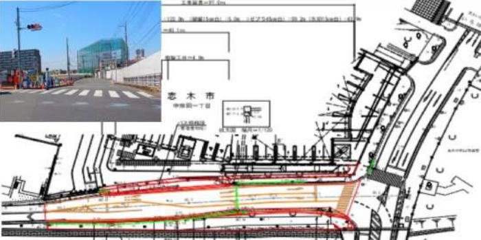
工事延長=97.0m 掘削工、舗装工、管渠工、街路工、区画線工、緑石工など
